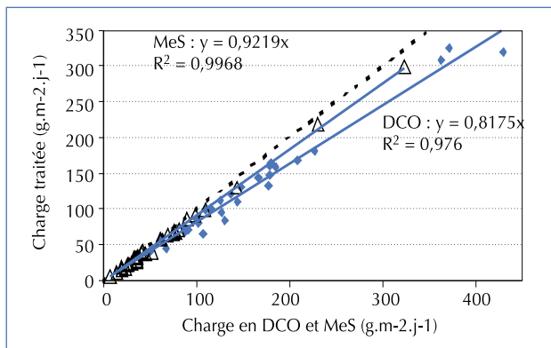
▲ Figure 4 – DCO et MeS traitées pour des concentrations en DCO d'entrée entre 520\text{-}1\ 400 \text{ mg} \cdot \text{l}^{-1} ; 0,15 < \text{CH} < 0,6 \text{ m} \cdot \text{j}^{-1} .
