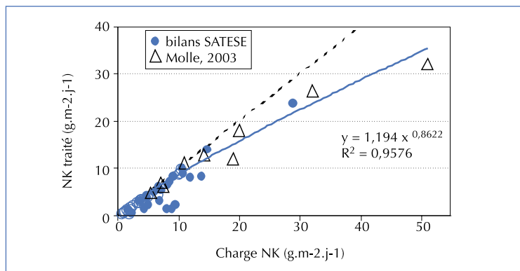
▲ Figure 8 – NK traité au 2 e étage (0,05 < CH < 2,2 m.j -1 ).
