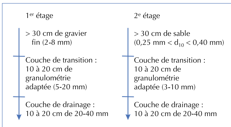
Figure 2 – Profils granulométriques.
